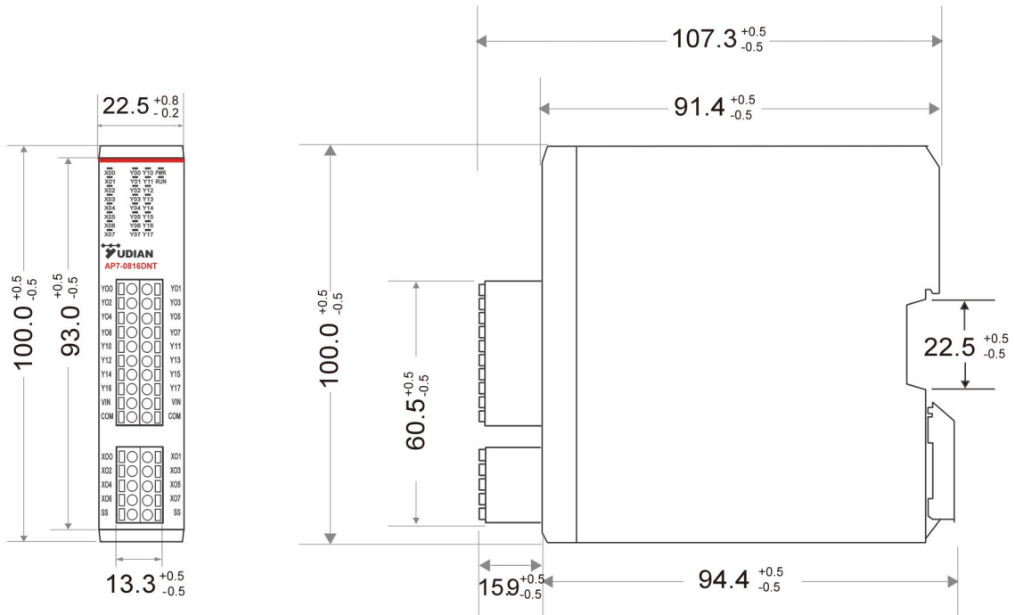
主视图
