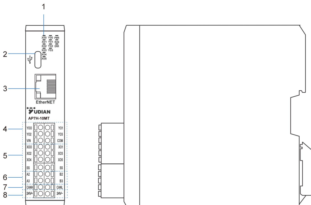
AP7H-10MT PLC 接口示意图
