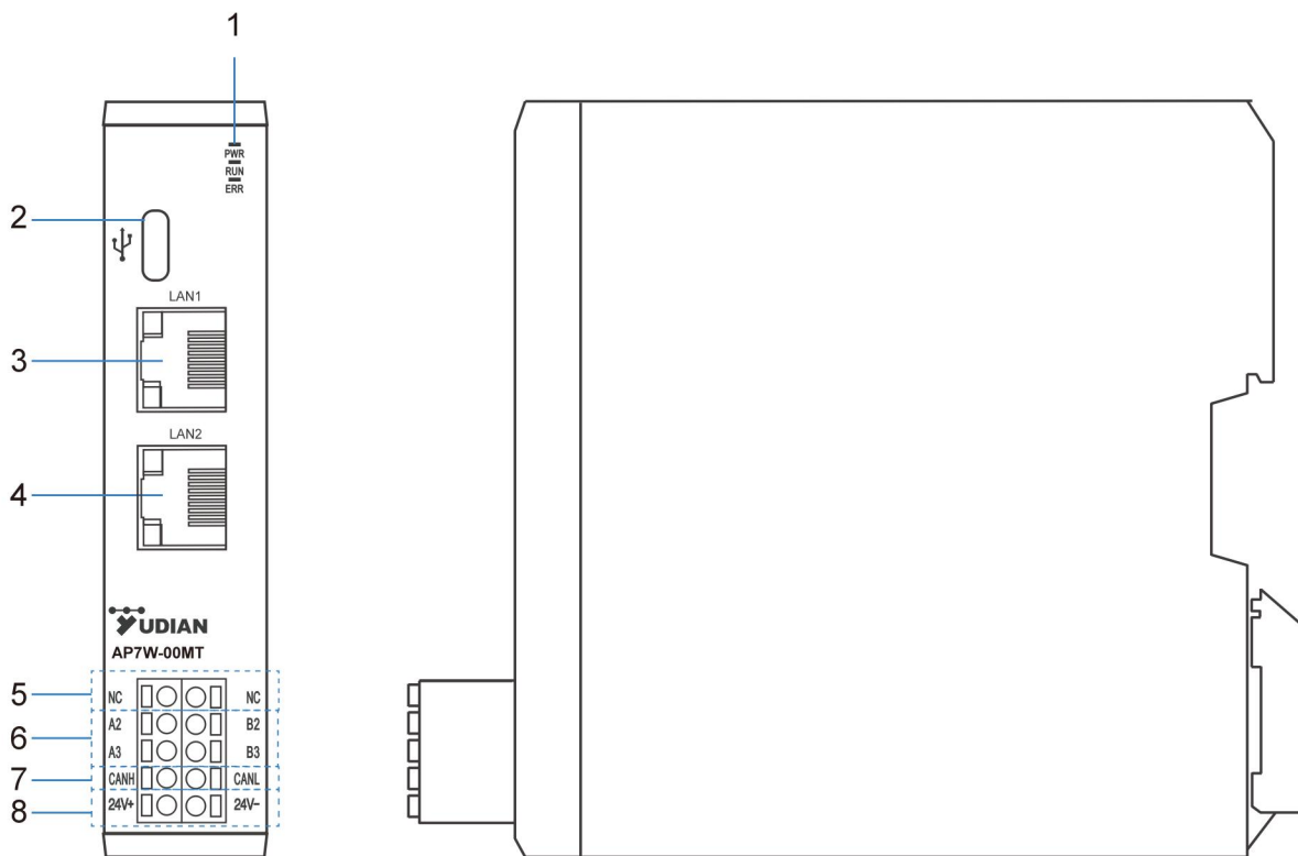
AP7W-00MT PLC 接口示意图
